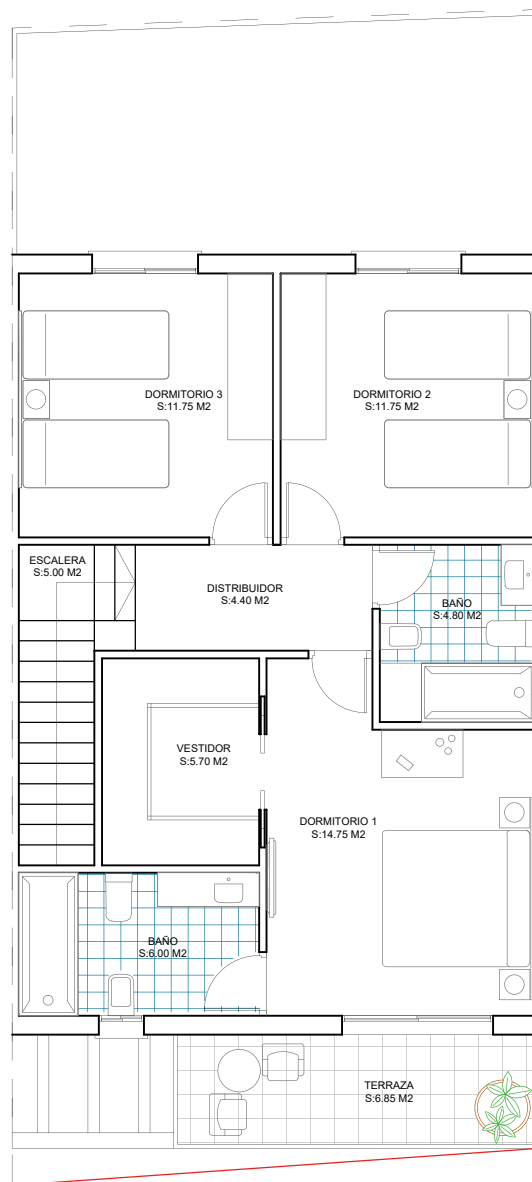
PLANTA 1º
